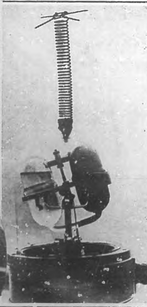
Aparato lumínico operado por medio de la electricidad, que posee el faro construido en Hartlepool y que hace innecesarios los servicios del torrero.
